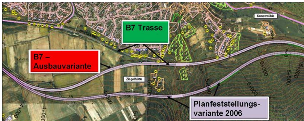
Abb. 10: Trassenvarianten für den Neubau der BAB A 44 zwischen Kaufungen und Helsa (Planfeststellungsentwurf 2006 und Ausbau der bestehenden B 7 nach den Planungen im Jahr 2010)
